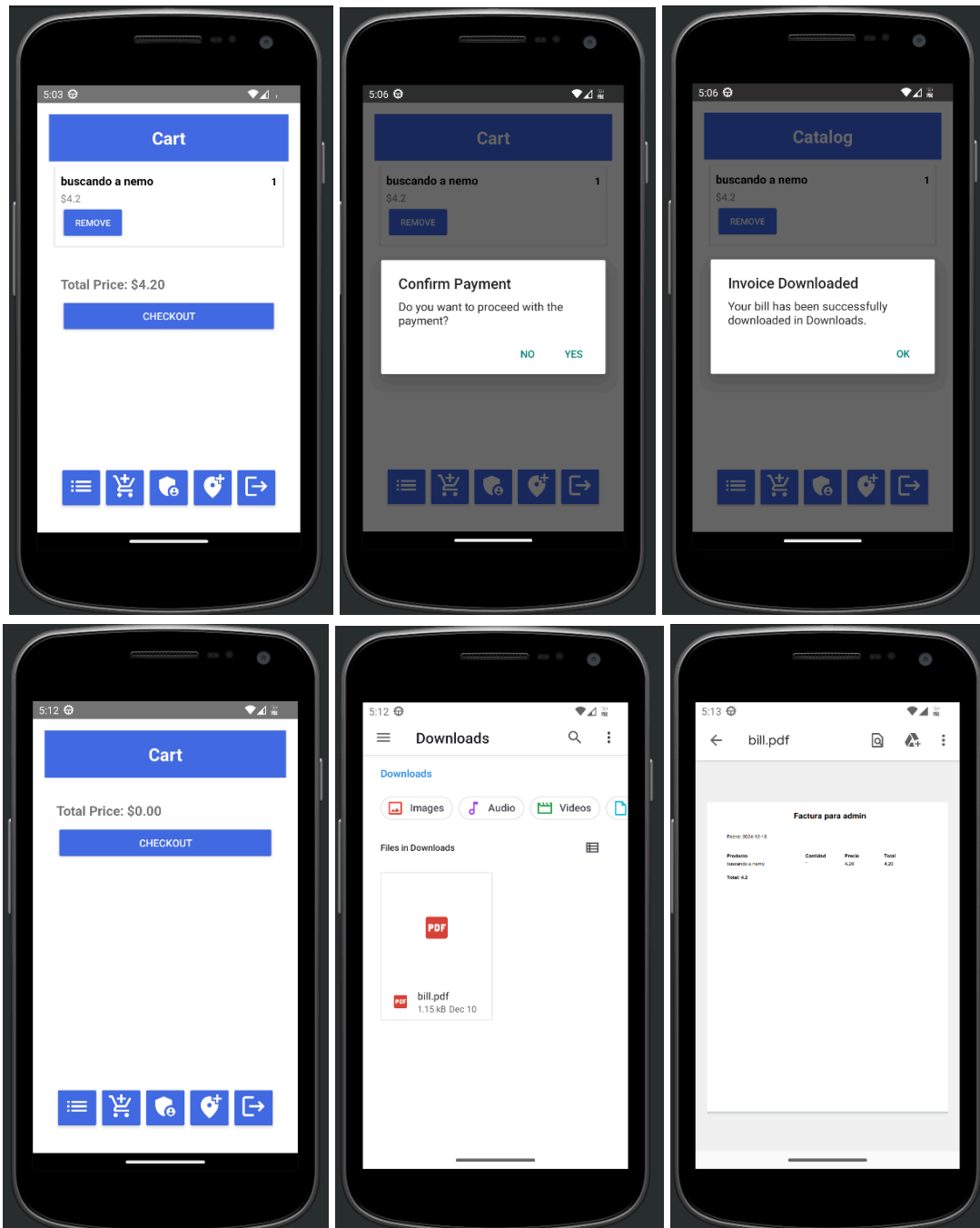
Figura 4. Pruebas de la realización de la compra
